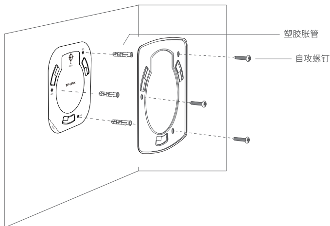
图3-10 固定安装架到墙面示意图
